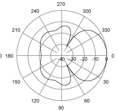
H-Plane | 146 MHz
